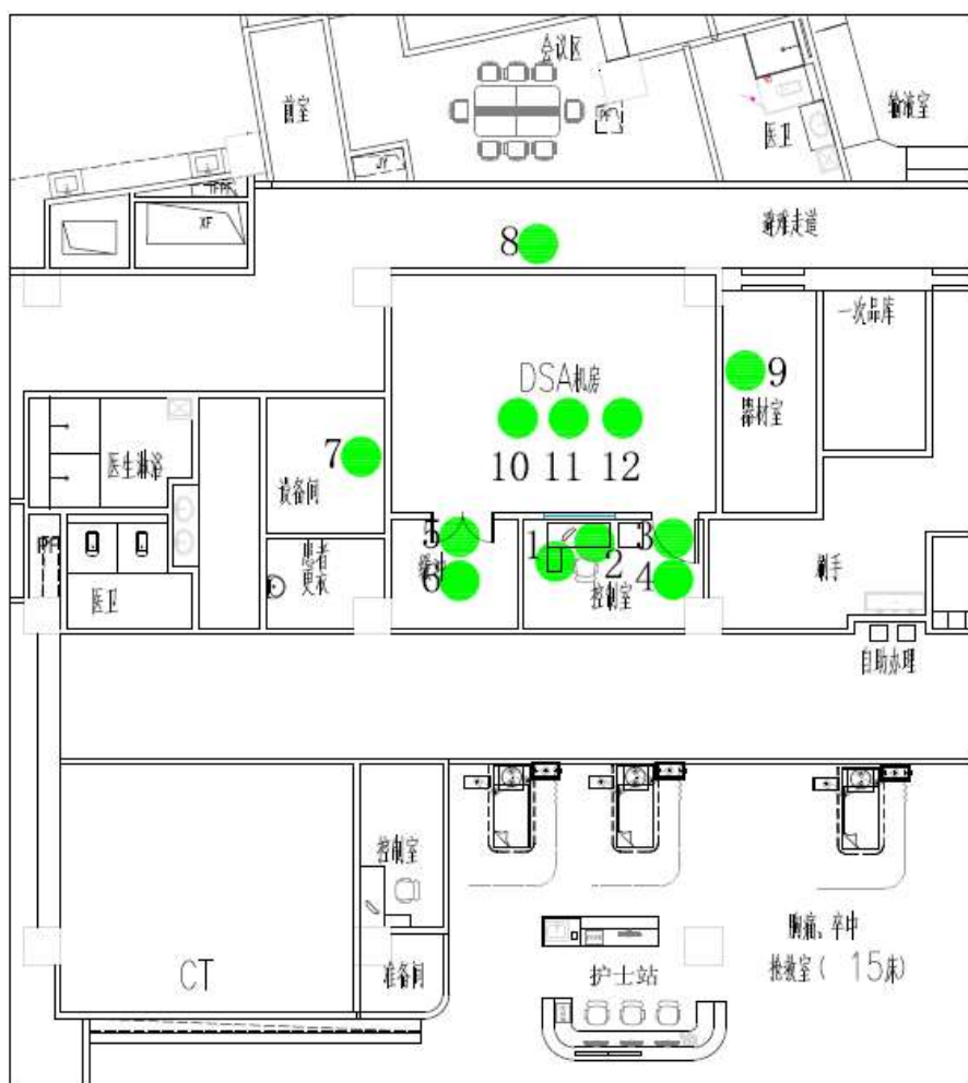
图 6-2 一层 DSA 机房监测点位示意图
