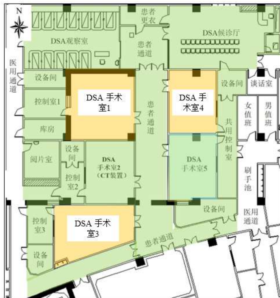
附图三 负一层放射科 DSA 机房周边布局图
