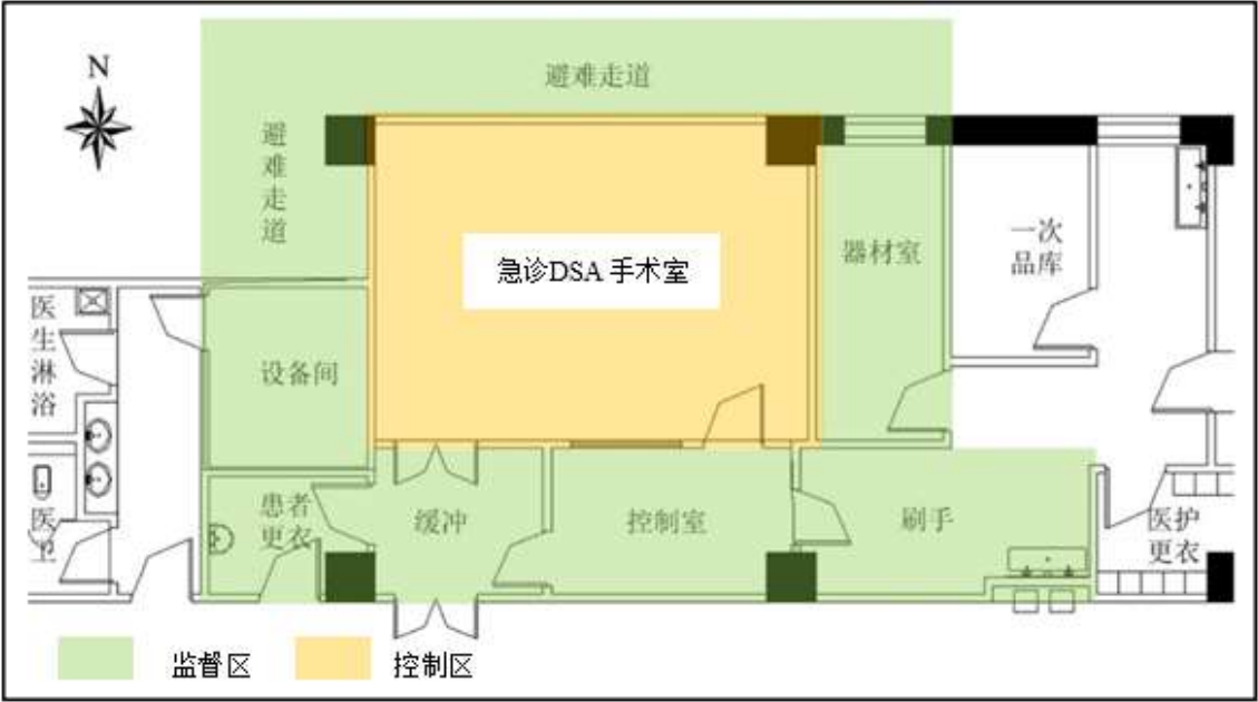
图 3-1 一层急诊 DSA 机房区域的控制区与监督区划分
