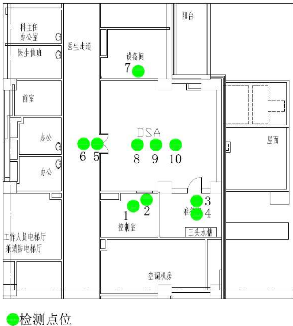
图 6-3 七层 DSA 机房监测点位示意图
