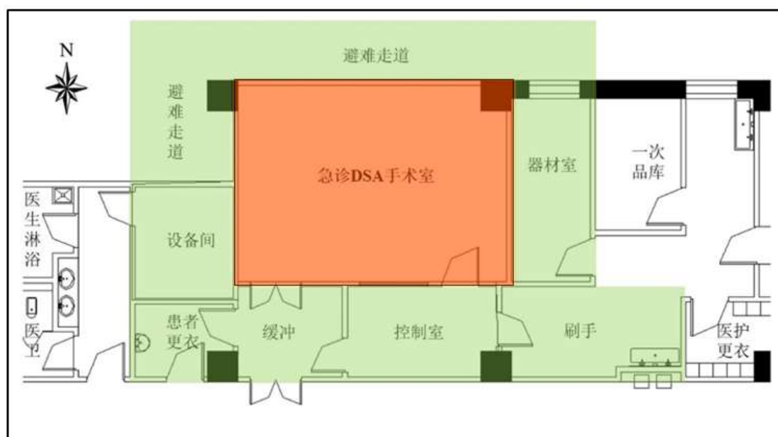
附图四 一层急诊 DSA 机房周边布局图
