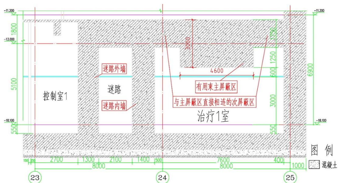
5b) 治疗 1 室 B-B 剖面图
