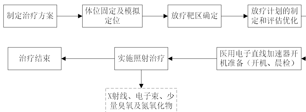
图 2-2 医用电子直线加速器工作流程及产污环节示意图
