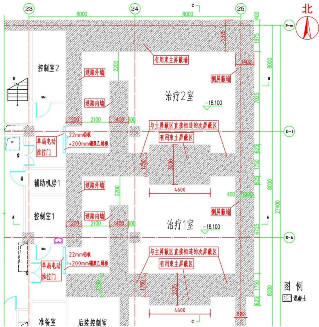
5a) 治疗 2 室、治疗 1 室平面布置图
