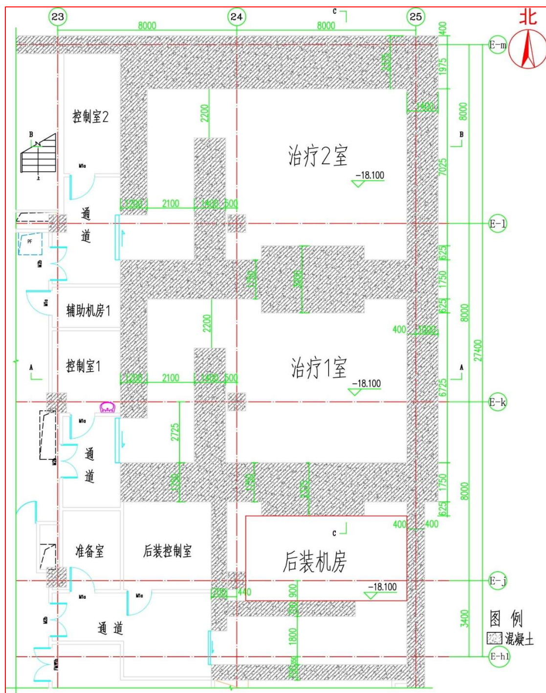
附图三 治疗室及后装机平面布置图
