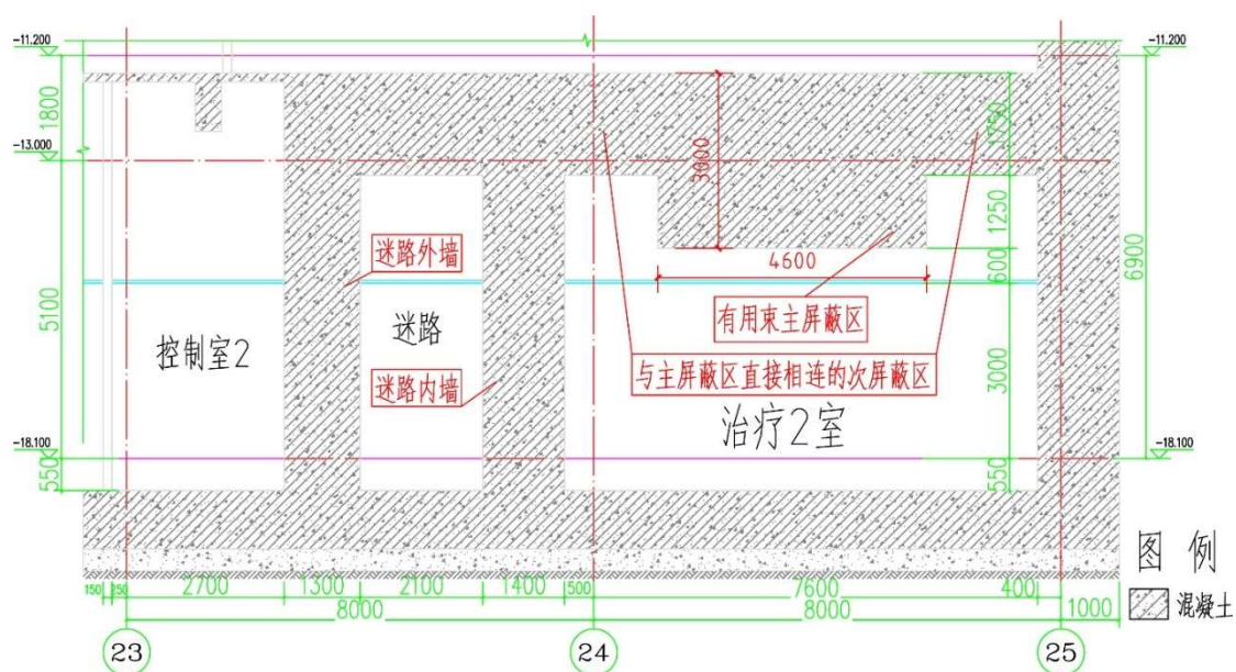
5c) 治疗 2 室 A-A 剖面图
